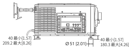
俯视图
