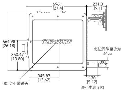
侧视图
