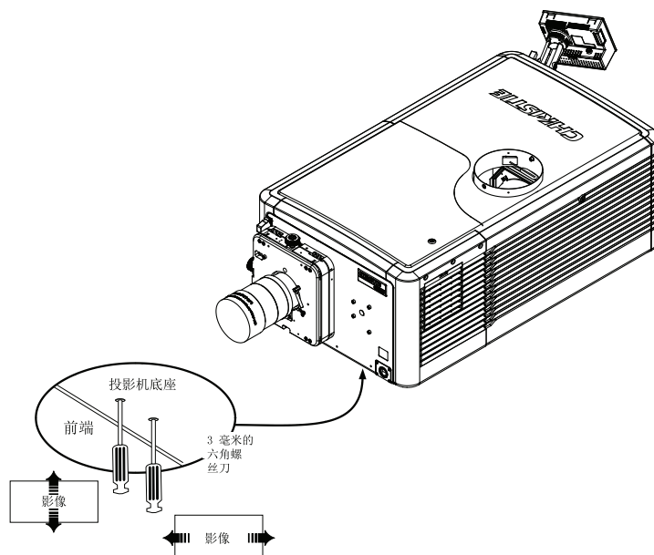
图 2-25 折叠式反射镜调整
