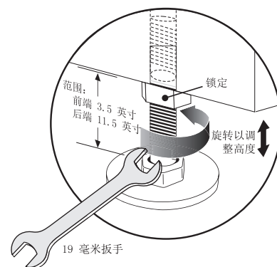
图 2-2 调整支脚
