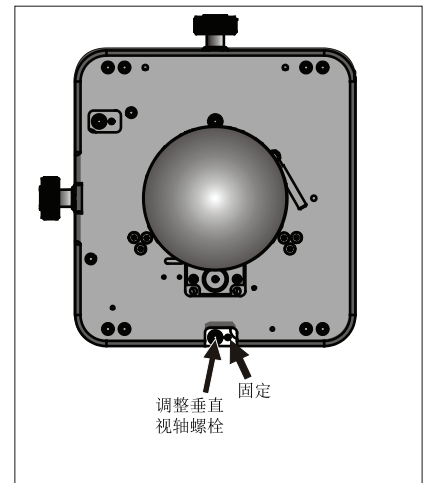
图 2-24 调整垂直观轴螺栓
