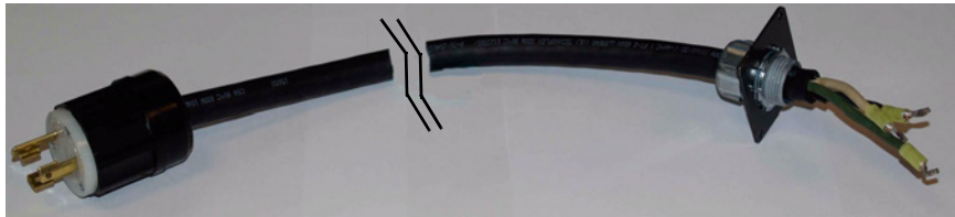
图 2-13 Nema-L630A 250V 电源插头 (116-102104-01) 实际长度 1.5 米
