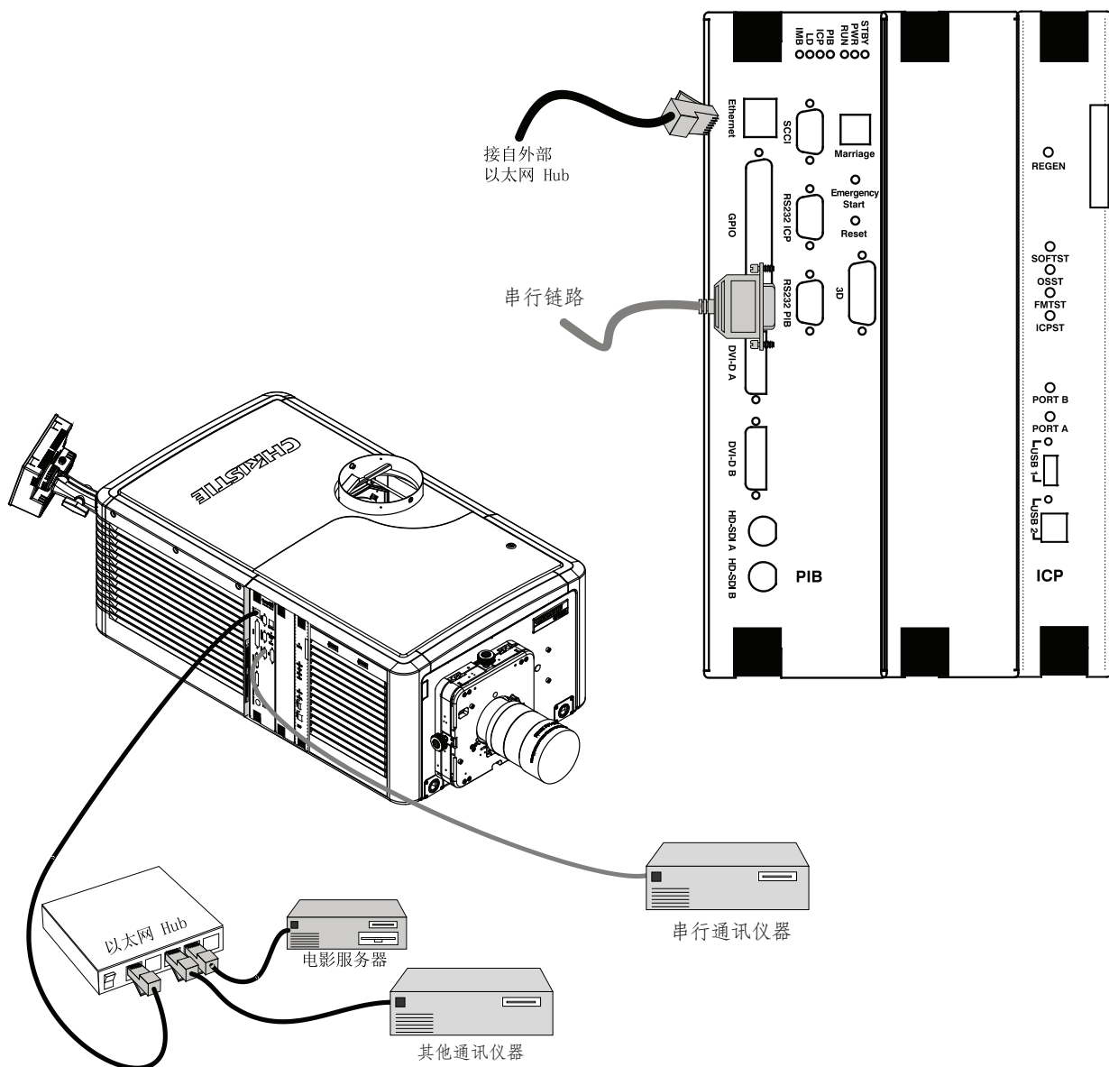
图 2-16 通讯连接
