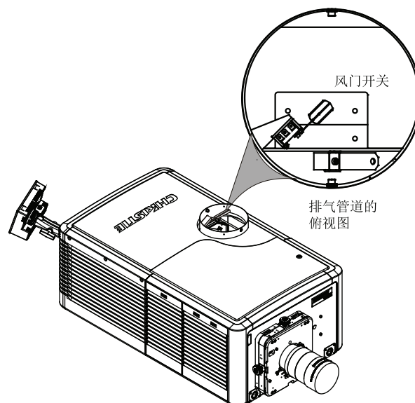
图 2-6 排气管道风门开关
