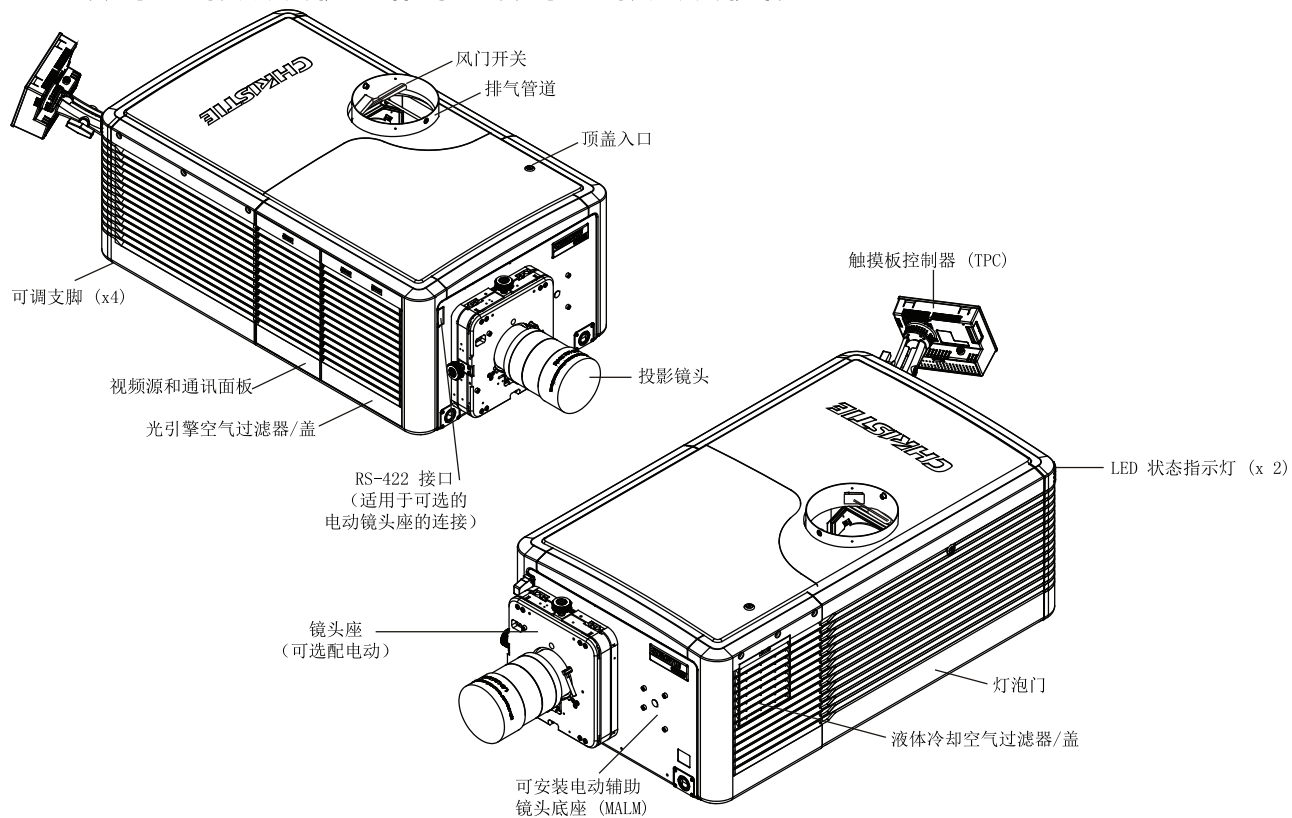
图 1-1 数字电影放映机概述
