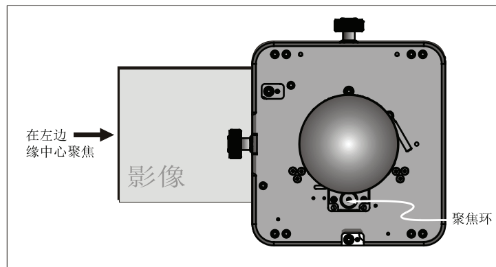
图 2-20 调整聚焦
