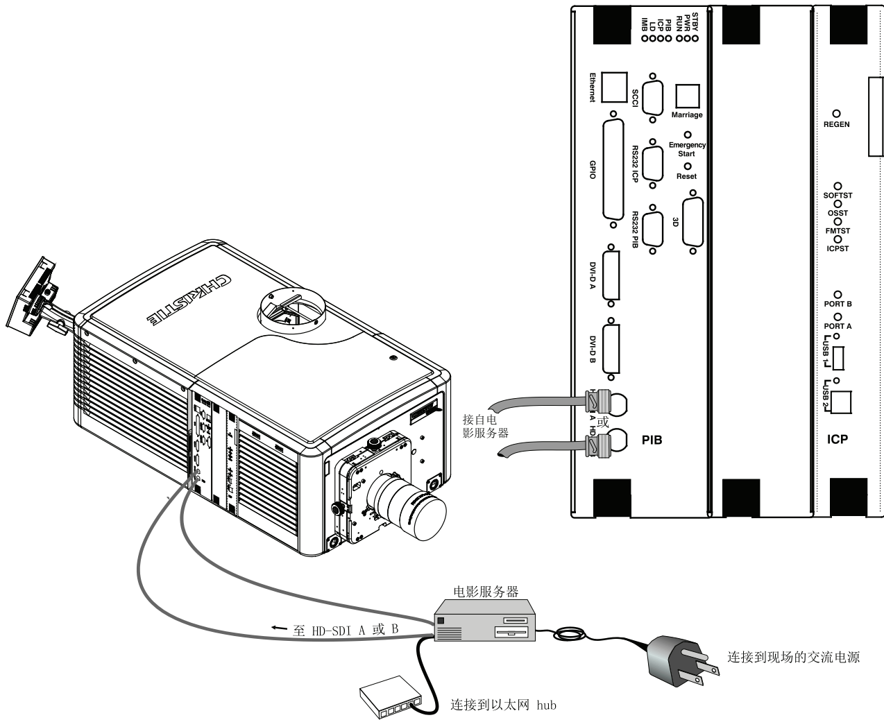
图 2-15 连接电影视频源
