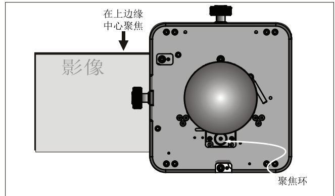
图 2-23 聚焦屏幕顶部中心位置
