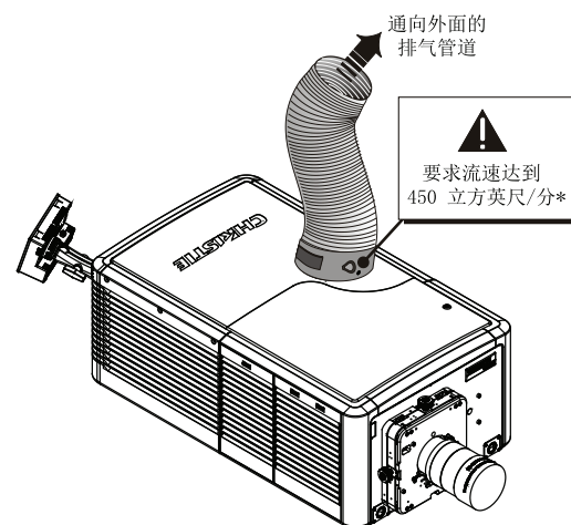
图 2-5 连接排气管道
