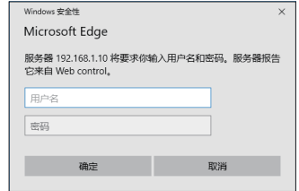
登录窗口
