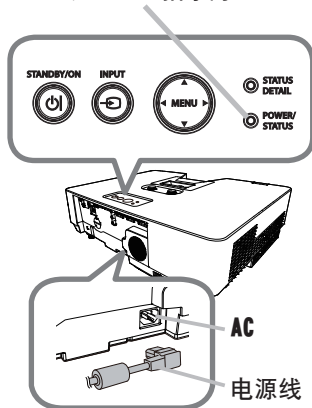
POWER/STATUS 指示灯
