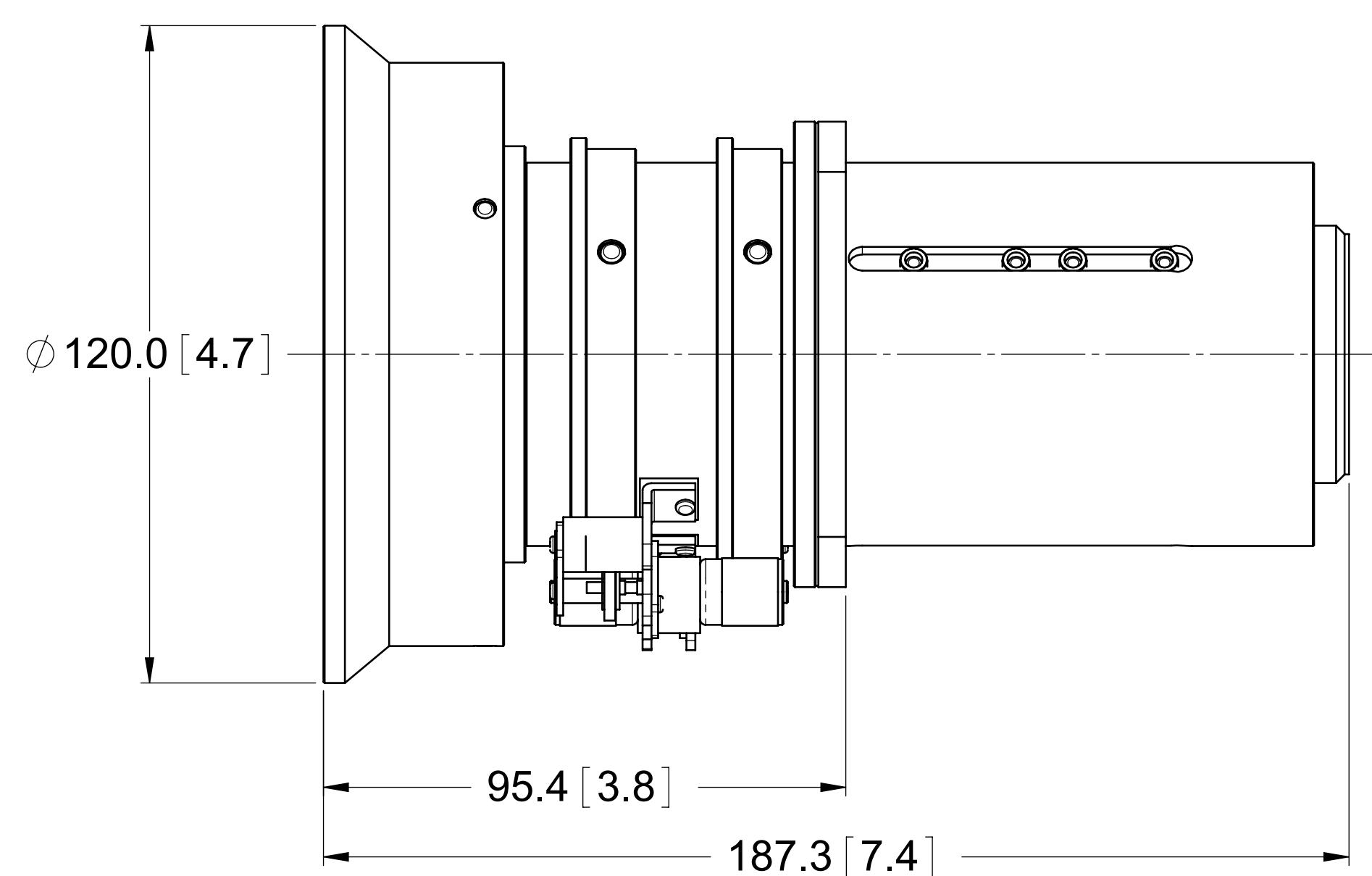
133-102104-XX 1.5-2.0:1 ZOOM
