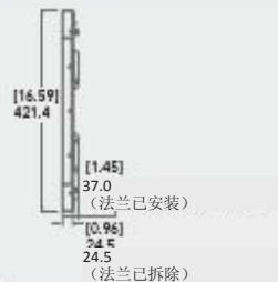
3x1基座套件侧视图
